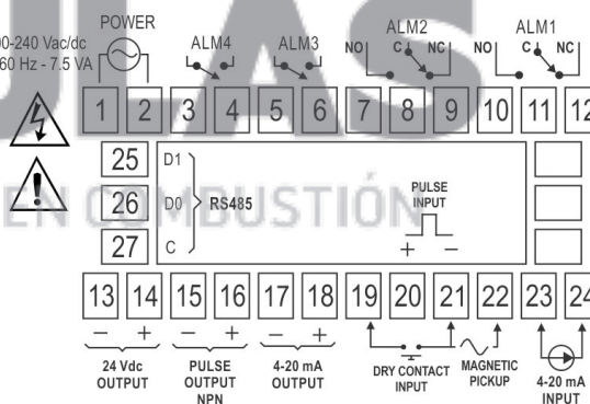
Fig. 1 - Bornes de conexión del panel trasero
