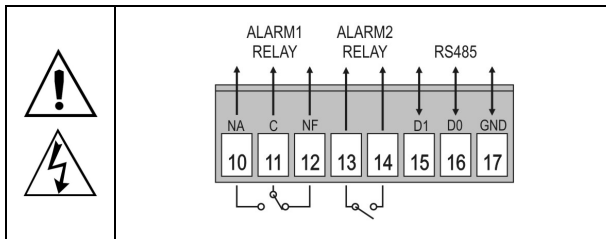
Figura 02 - Conexiones de alarmas y comunicación serial
