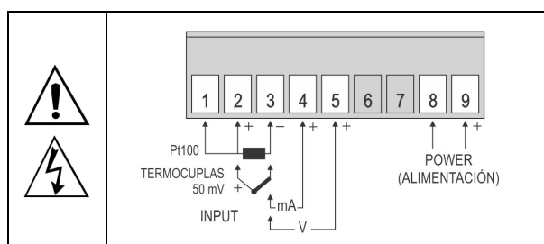
Figura 01 - Conexiones de las entradas y alimentación
