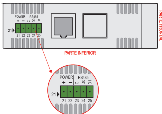
Figura 09 – Conexión de la interfaz RS485
