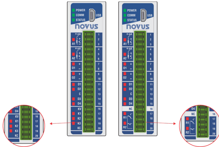
Figura 17 – Salidas digitales
