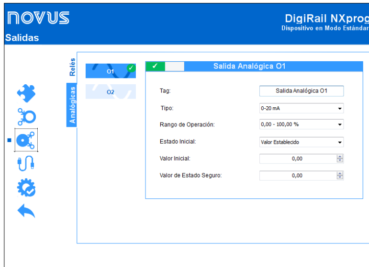
Figura 30 – Salidas Analógicas
