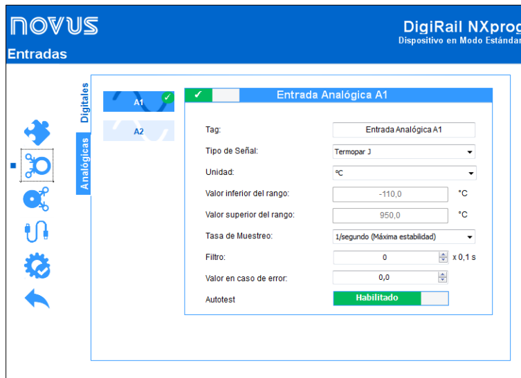
Figura 28 – Entradas Analógicas
