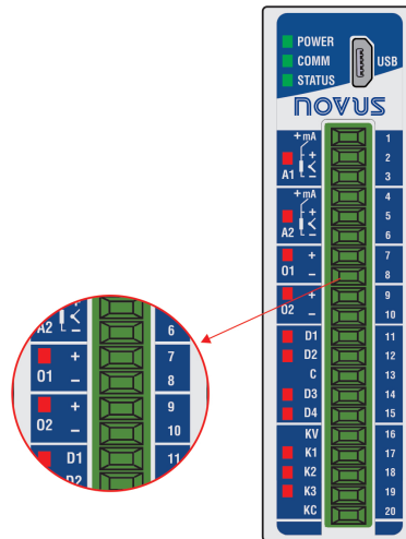
Figura 15 – Salidas analógicas
