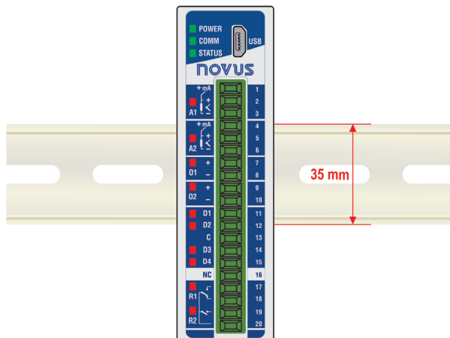
Figura 05 – Instalación mecánica
