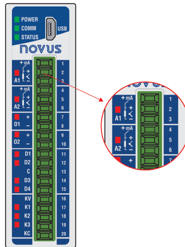
Figura 11 – Entradas analógicas
