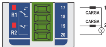
Figura 23 – Relé
