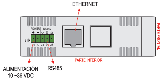
Figura 07 – Conexiones de alimentación y puertos de comunicación
